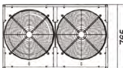
Вид сверху
